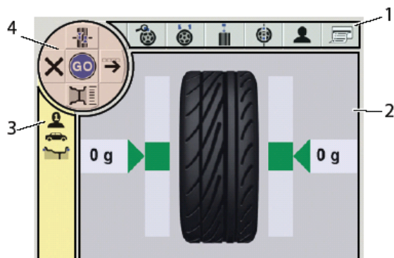
4. ábra: Kiegyensúlyozási főképernyő
