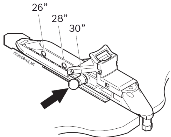
3. ábra: A mozgatható vezető sínek beállítása
